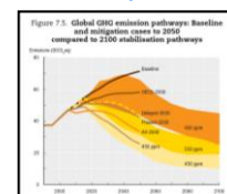
[7.5. sz. ábra] Globális üvegházhatású gázkibocsátási folyamatok: Bázisvonal és enyhítési esetek 2050-ig a 2100-es stabilizációs folyamatokhoz viszonyítva 1
